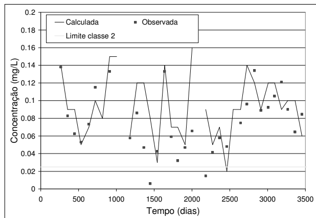
Figura 10 - Ajuste dos fosfatos totais no TA 004 (foz do Taquari)
