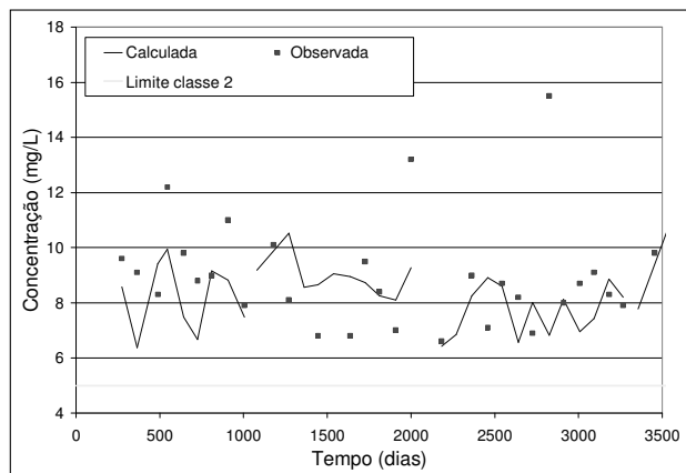
Figura 11 - Ajuste do oxigênio dissolvido no TA 451 (Bom Jesus)
