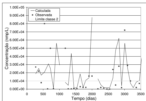
Figura 12. Ajuste dos coliformes fecais no TA 275 (Nova Roma do Sul/Nova Pádua)
