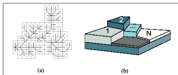
Figura 2 - Subdivisão de uma bacia em células ligadas por linhas que representam a rede de drenagem e da célula em n blocos, de acordo com o uso do solo (Collischonn, 2001)
