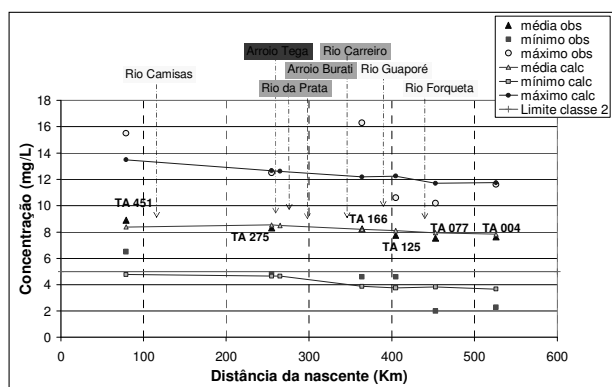
Figura 13 - Valores médio, máximos e mínimos de concentração de OD ao longo do curso do Taquari-Antas no período de 1993 a 2002
