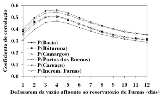
Figura 3 - Coeficiente de correlação entre diferentes variáveis (precipitação média diária nas sub-bacias de montante e na bacia de montante de Furnas) e a vazão afluente ao reservatório de Furnas com defasagens de um a doze dias.
