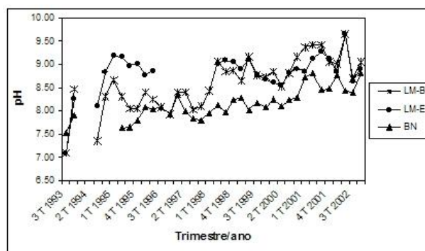
Figura 5 - Gráfico das séries históricas das médias trimestrais e gráfico das médias dos trimestres das medições de pH - pontos LM-B, LM-E e BN.
