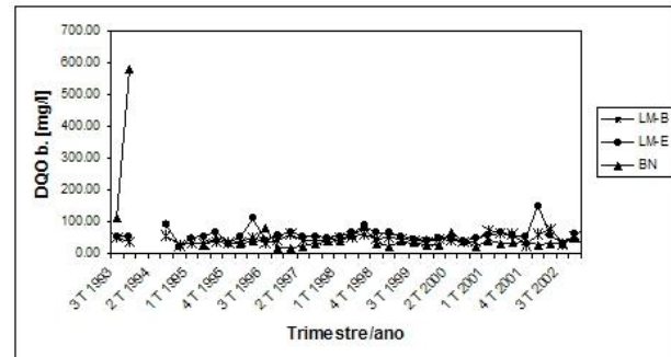
Figura 11 - Gráfico das séries históricas das médias trimestrais e gráfico das médias dos trimestres das medições de DQO b. - pontos LM-B, LM-E e BN.
