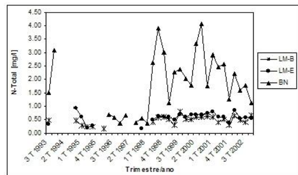
Figura 12 - Gráfico das séries históricas das médias trimestrais e gráfico das médias dos trimestres das medições de N-Total - pontos LM-B, LM-E e BN.
