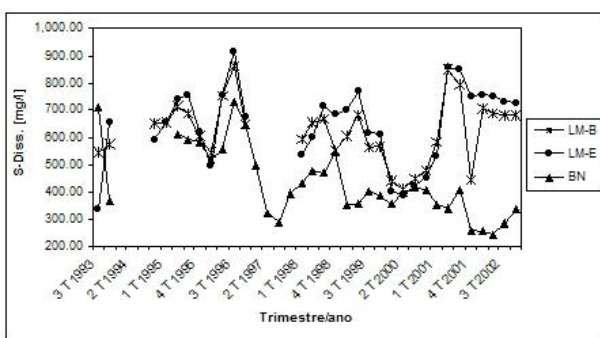
Figura 9 - Gráfico das séries históricas das médias trimestrais e gráfico das médias dos trimestres das medições de S-Diss. - pontos LM-B, LM-E e BN.
