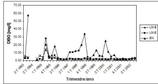
Figura 10 - Gráfico das séries históricas das médias trimestrais e gráfico das médias dos trimestres das medições de DBO - pontos LM-B, LM-E e BN.
