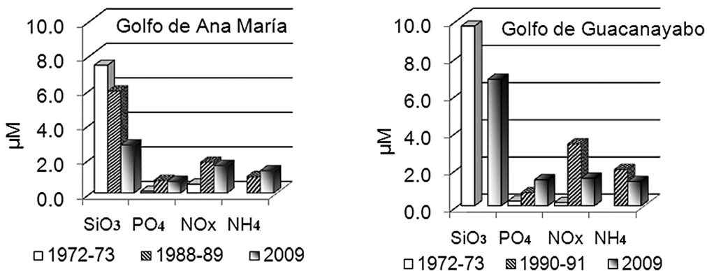
Fig. 5. Concentración media de nutrientes en los golfos de Ana María y Guacanayabo en tres periodos diferentes
