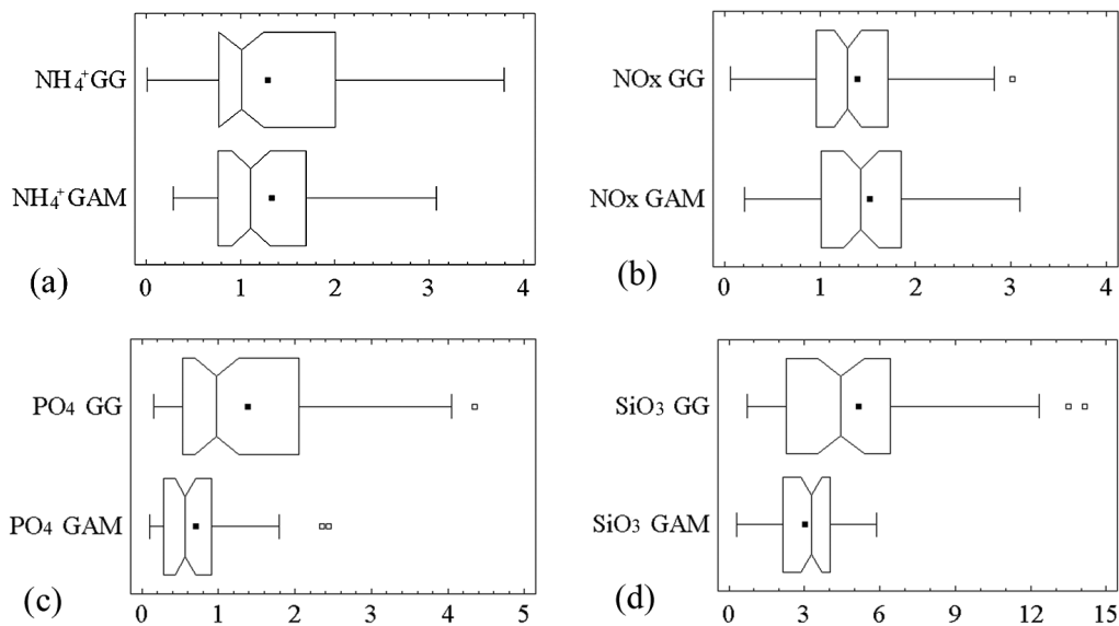
Fig. 2. Análisis comparativo de los nutrientes entre los golfos Guacanayabo (GG) y Ana María (GAM). Resultado de la prueba de Mann-Whitney (Wilcoxon), nivel de confianza del 95%
