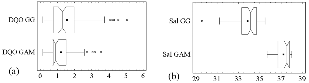
Fig. 3. Análisis comparativo de la DQO y la salinidad entre los golfos Guacanayabo (GG) y Ana María (GAM). Resultado de la prueba de Mann-Whitney (Wilcoxon), nivel de confianza del 95% Fig. 3. Comparative analysis of COD and salinity between the Gulfs of Guacanayabo (GG) and Ana María (GAM). Results of Mann-Whitney (Wilcoxon) test, 95% confidence level
