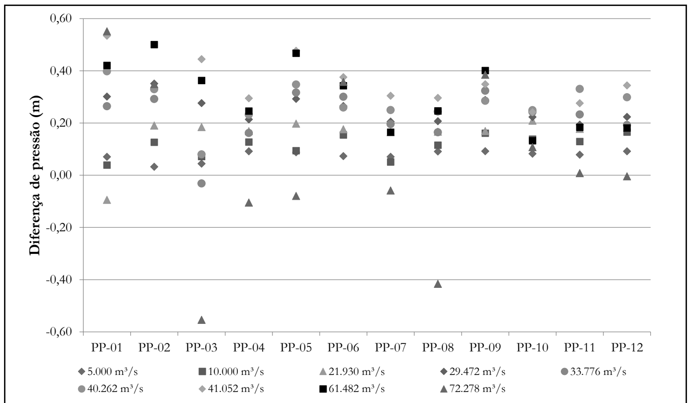
Figura 13 - Diferença nas medições dos piezômetros localizados no pilar
