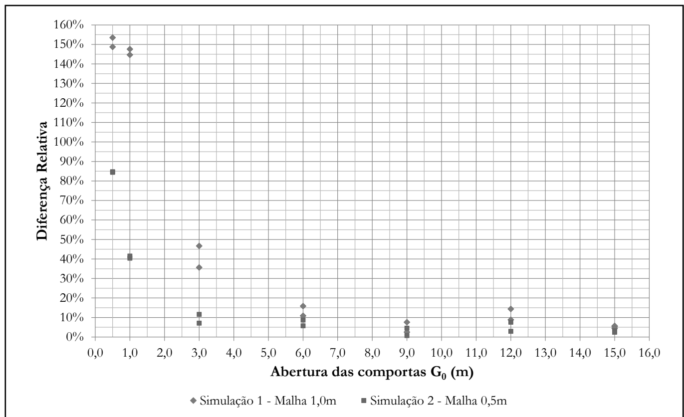
Figura 15 - Erro nas vazões simuladas para as duas malhas e diversas aberturas de comporta (ARAÚJO FILHO, 2014)
