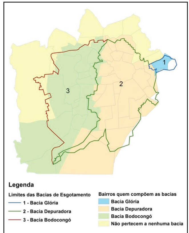
Figura 2 - Bacias de esgotamento da cidade de Campina Grande Fonte: Adaptado da CAGEPA (2014)
