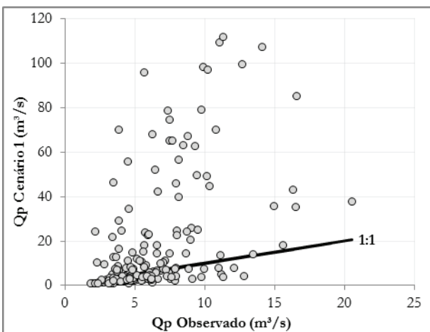
Figura 12 – Vazão de pico do cenário 1 versus observada
