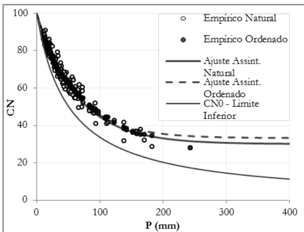
Figura 2 – Ajuste do modelo assintótico padrão aos dados da bacia
