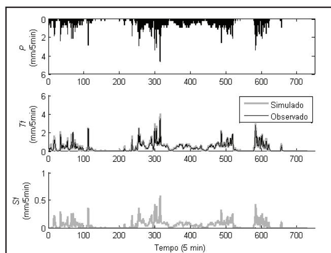
Figura 10 – Simulação do modelo de Rutter de chuva interna ( T_f ) e escoamento pelos troncos ( S_f ) para o maior evento (n°35), chuva externa ( P ) de 326 mm com o valor de Nash de 0,85
