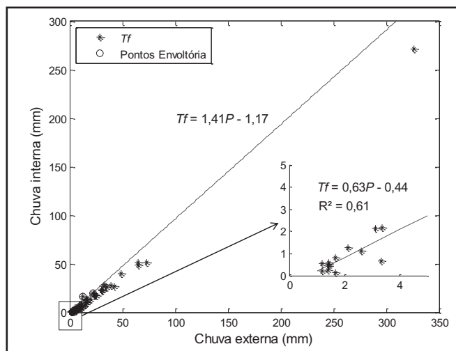
Figura 7 – Relação entre chuva externa e chuva interna. No gráfico menor é apresentada a relação entre P e Tf para eventos abaixo do ponto de inflexão (P<5mm)
