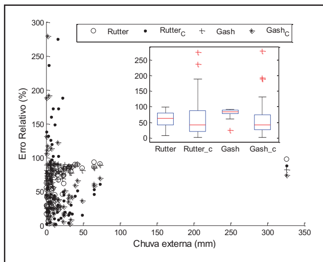
Figura 11 – Erro relativo para a I acumulada por evento pelo modelo de Gash e pelo modelo de Rutter e boxplot do erro relativo por evento dos dois modelos. GashC e RutterC é a simulação dos modelos utilizando os parâmetros de entrada calibrado
