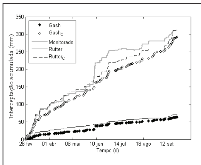
Figura 12 – Perda por interceptação acumulada monitorada, estimativa pelo modelo de Gash e estimativa pelo modelo de Rutter. GashC e RutterC é a simulação dos modelos utilizando os parâmetros de entrada calibrado
