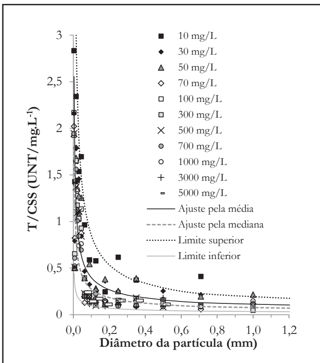
Figura 3 – Relação Turbidez/CSS para diferentes diâmetros da partícula de sedimento
