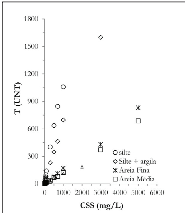
Figura 2- Relação entre a concentração de sedimentos suspensos (CSS) e a turbidez (T), considerando diferentes faixas granulométricas
