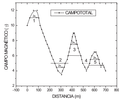
Figura 12 Gráfica representando la curva de campo magnético versus distancia (Anomalía AA*), del campo Petróleo-Química
