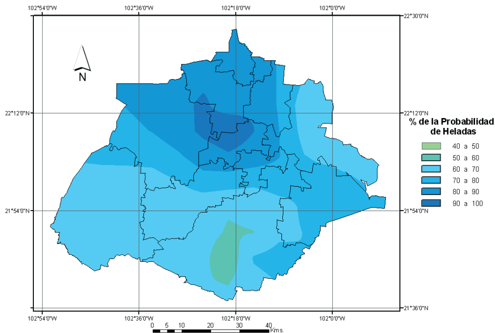
Figura 8. Probabilidad de ocurrencia de heladas en la primera decena de diciembre, periodo 1979-2001.
