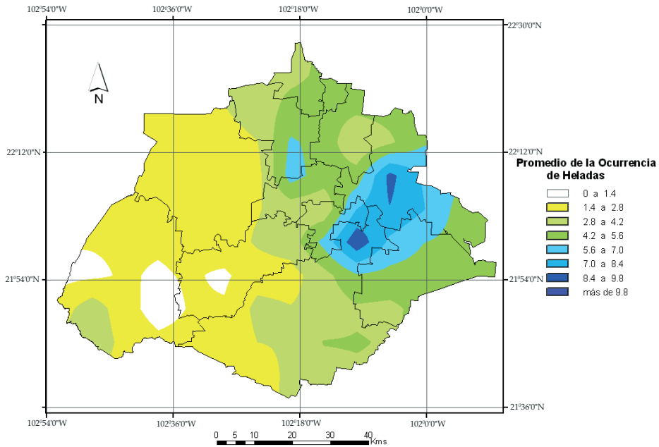
Figura 2. Presencia e incidencia de heladas en el mes de diciembre, periodo 1979-2001.
