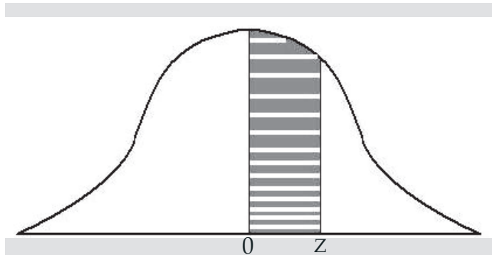
Figura 1. El lado sombreado de la gaussiana representa los valores positivo que se muestran en tablas (Ostle, 1979).
