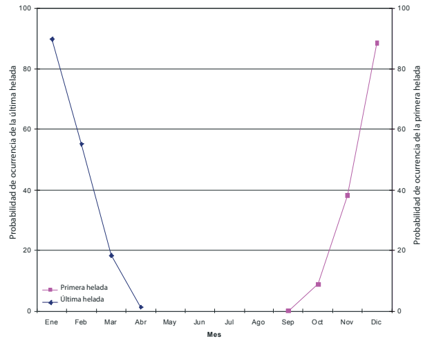
Figura 7. Probabilidad de ocurrencia de la primera y última helada en la estación San Bartolo, Ags., periodo 1979-2001.
