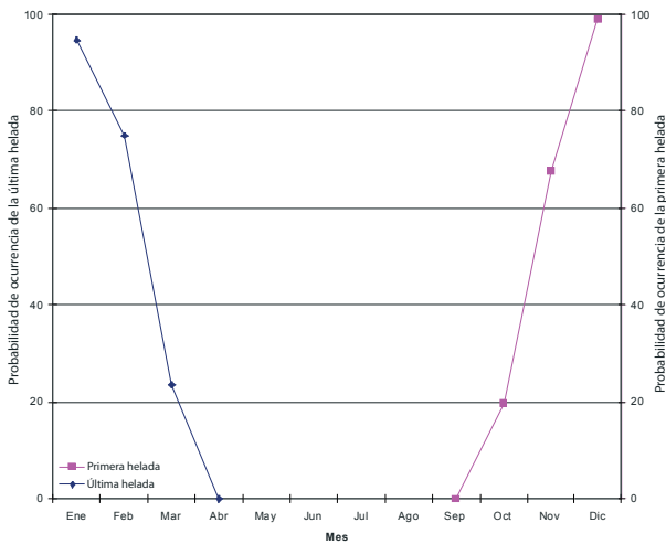
Figura 6. Probabilidad de ocurrencia de la primera y última helada en la estación Pabellón de Arteaga, Ags., periodo 1979-2001.
