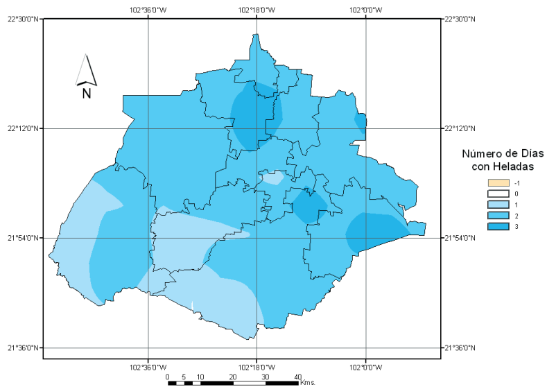
Figura 11. Anomalía en el número de días con heladas en condiciones normales para el mes de diciembre.
