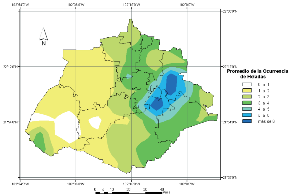
Figura 3. Presencia e incidencia de heladas en el mes de febrero, periodo 1979-2001.
