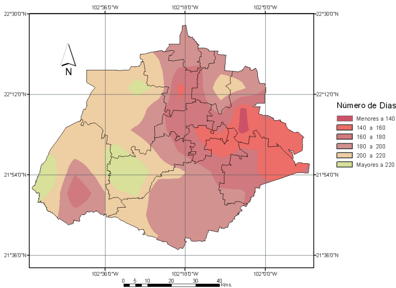
Figura 14. Número de días libres de heladas, condición El Niño fuerte , serie 1982, 1983, 1987, 1992, 1997 y 1998.
