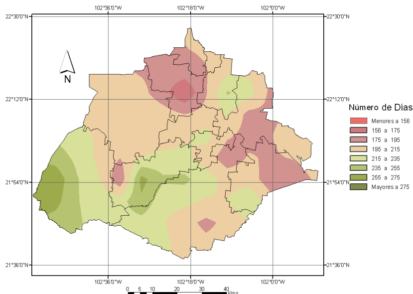
Figura 13. Número de días libres de heladas, condición climática, serie 1979 a 2001.
