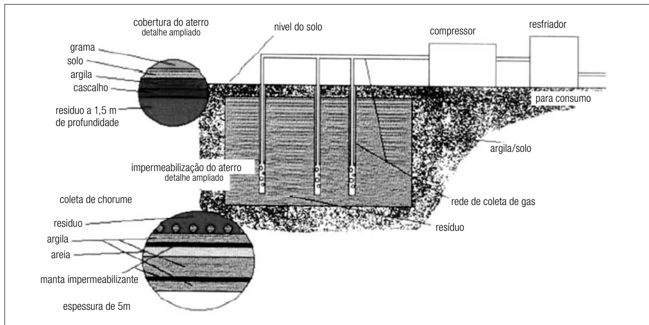
FIGURA 1. Esquema básico de um aterro sanitário com recuperação de biogás
