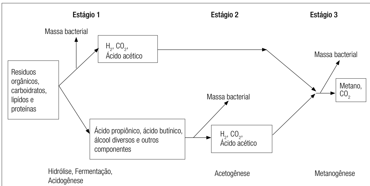
FIGURA 2. ETAPAS do processo de produção do biogás.
