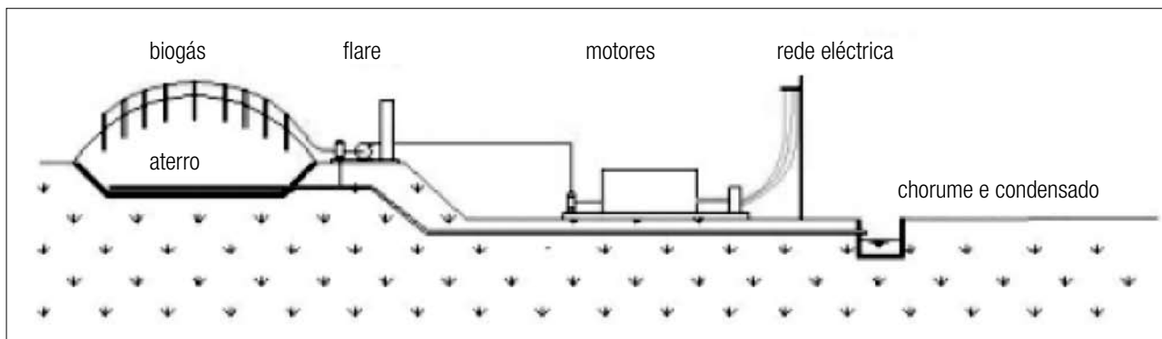
FIGURA 3. Esquema ilustrativo da produção de biogás de aterro.
