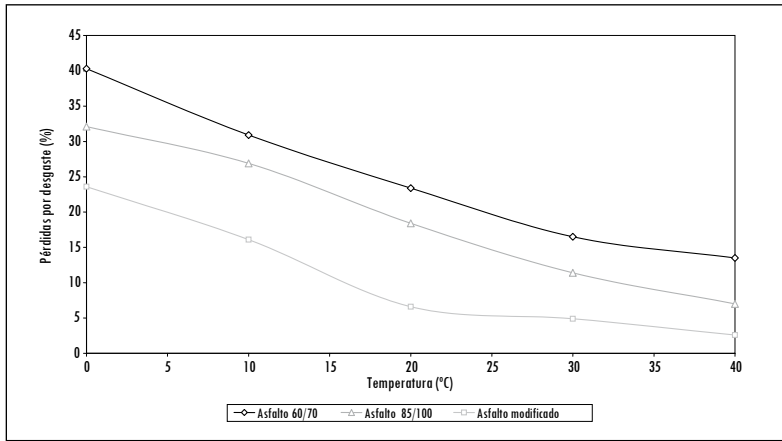
Figura 13. Influencia de la temperatura en la cohesión para las muestras con granulometría md12 en estado húmedo
