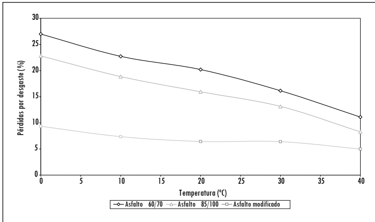
Figura 10. Influencia de la temperatura en la cohesión para las muestras con granulometría md10 en estado seco
