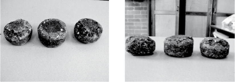
Figura 3. Estado de las muestras UCL después de ensayadas
