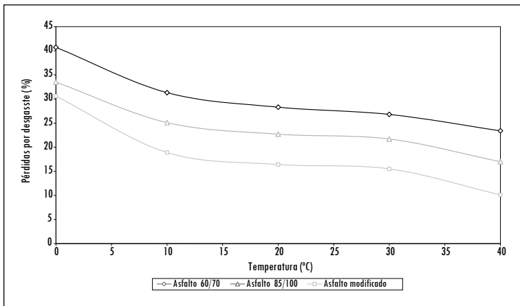
Figura 11. Influencia de la temperatura en la cohesión para las muestras con granulometría md10 en estado húmedo
