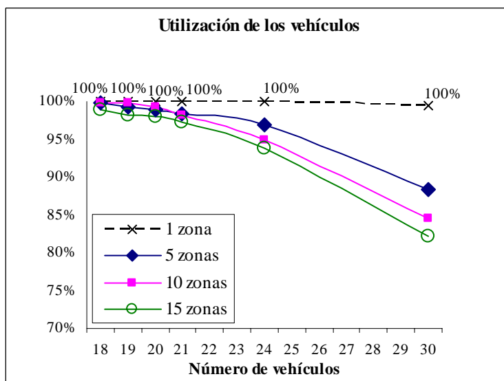
Figura 6. Resultados de simulación para el nivel de utilización de los vehículos
