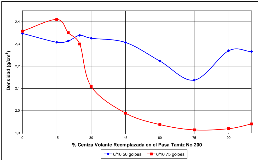
Figura 4. Variación de la densidad con respecto al reemplazo de ceniza en el tamiz pasa número 200
