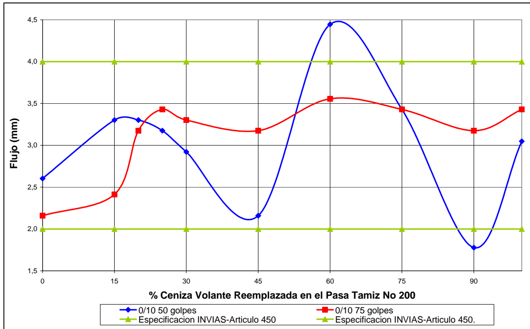
Figura 5. Variación del flujo con respecto al reemplazo de ceniza en el tamiz pasa número 200
