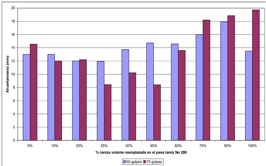
Figura 7. Ahuellamiento con respecto al reemplazo de ceniza volante
