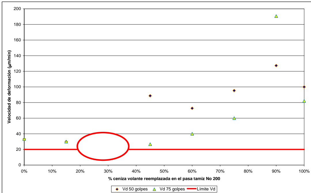
Figura 8. Velocidad de deformación medida en cada porcentaje de reemplazo de ceniza volante
