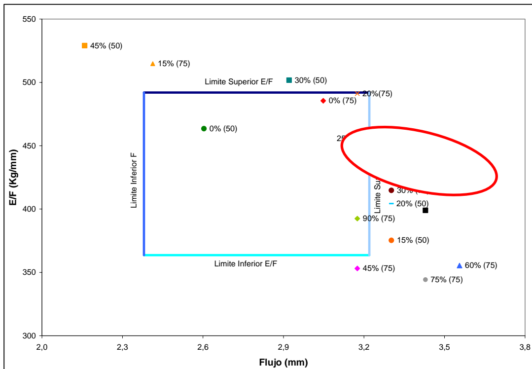
Figura 6. Variación de la relación estabilidad-flujo
