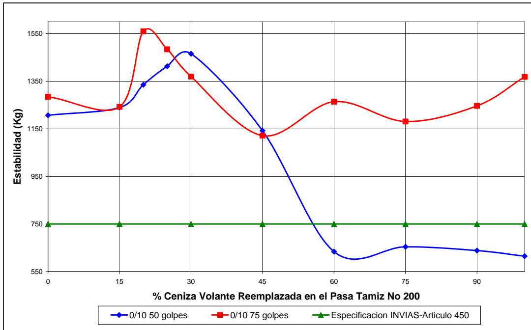
Figura 3. Variación de la estabilidad con respecto al reemplazo de ceniza en el tamiz pasa número 200
