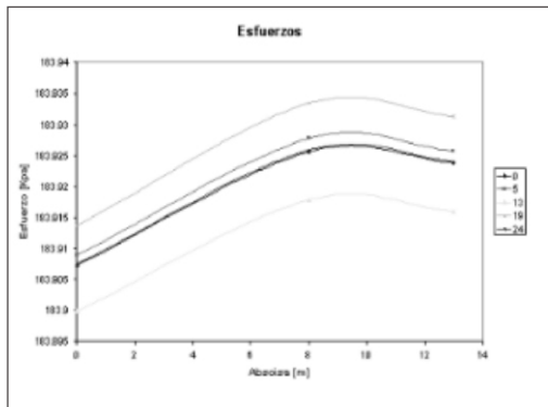
Figura 7. Esfuerzos bajo cada una de las zapatas a una profundidad de 0.5 m.
