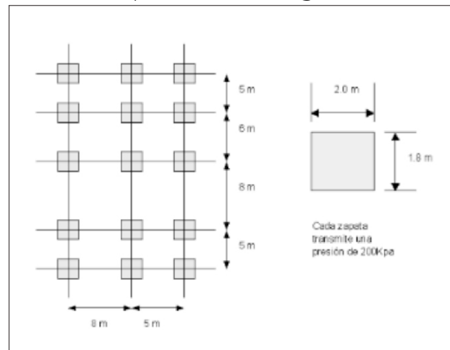
Figura 5. Geometría del problema
