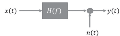
Figura 1. Representación de un sistema lti para un canal plc.
