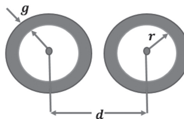
Figura 12. Sección transversal de una línea bifilar asociada al cableado eléctrico en ambientes residenciales
