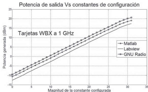
FIGURA 8. Resultados de las pruebas de caracterización: Potencia de salida vs Constantes de configuración.
