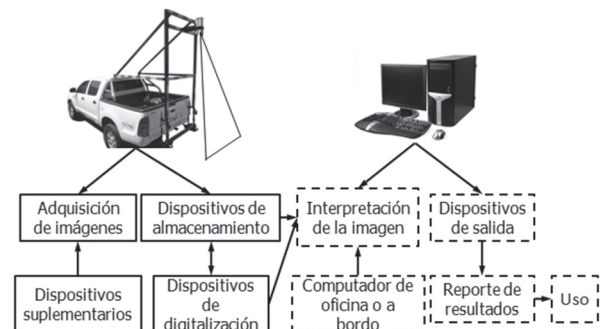
FIGURA 13. Elementos de un sistema de inspección de pavimentos por imágenes
