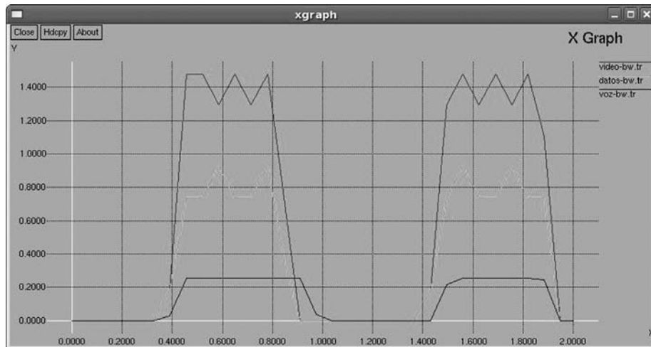
FIGURA 4. Throughput para el evento de 3 fallas en los enlaces sin aplicar mecanismos de recuperación (caso 1).
