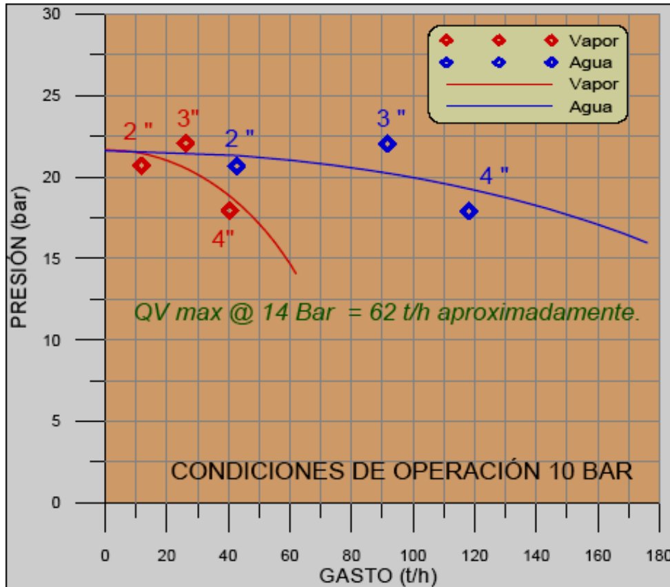
Fig. 2. Curva característica de producción del pozo Az-68D después de su estimulación ácida.
