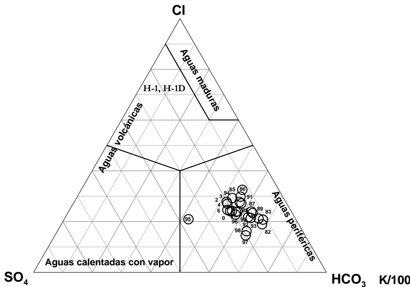
Fig. 5. Contenido relativo de Cl-SO 4 -HCO 3 de los pozos H-1 y H-1D del campo geotérmico de Los Humeros (Giggenbach, 1992).
