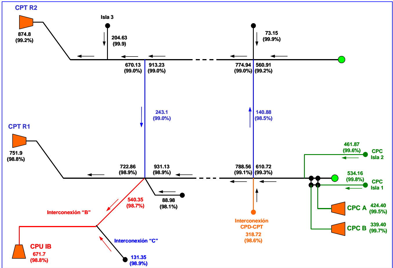
Fig. 4. Distribución de flujos en los principales ductos de CPT y CPC
