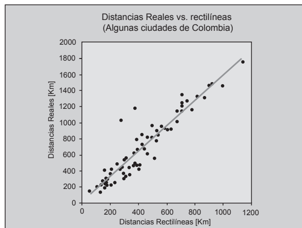
Figura 6. Distancias reales vs rectilíneas. Fuente: Vidal (2011). Optimización de cadenas de abastecimiento.
