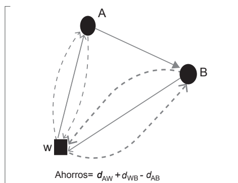
Figura 2. Principio básico del método de los ahorros. Fuente: Vidal (2011). Optimización de cadena de abastecimiento.
