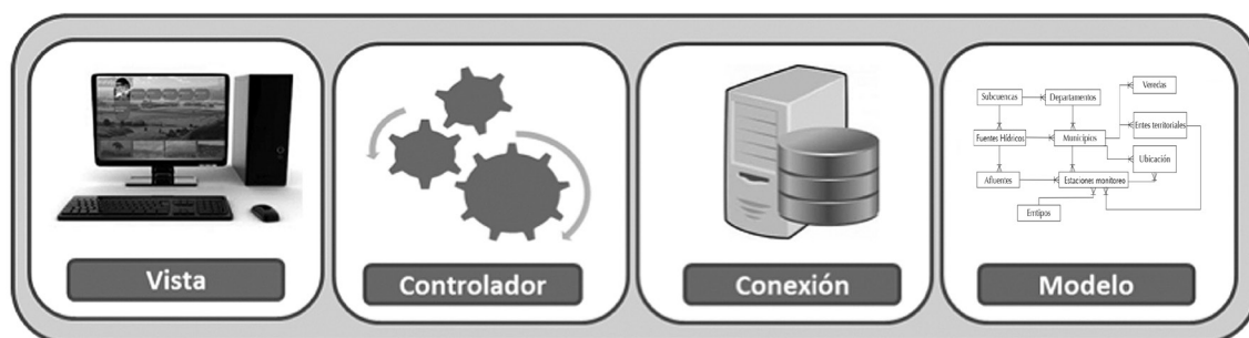
Figura 7. Arquitectura modelo-vista-controlador
