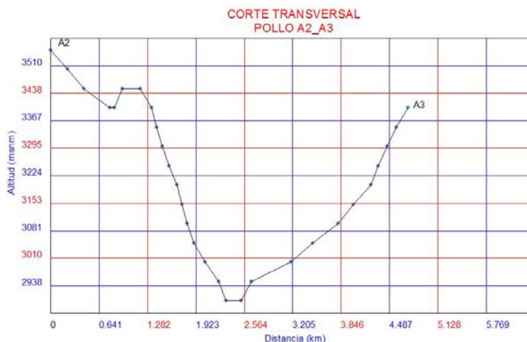
Figura 2. Perfil transversal de la Microcuenca Pollo.
