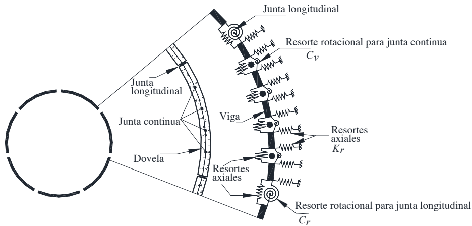
Fig. 4: Discretización estructural del modelo numérico.
