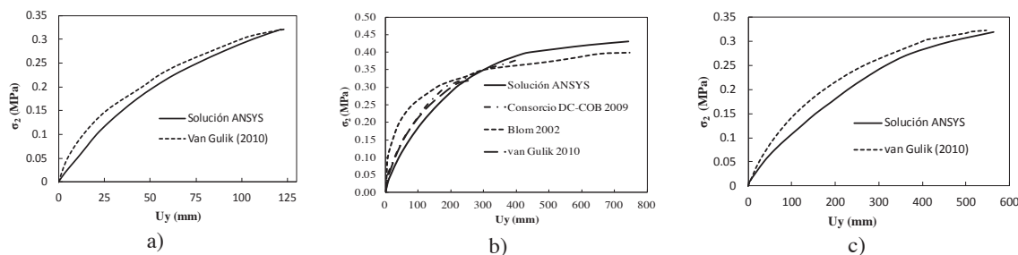
Fig. 15: a) Deformaci3n del anillo y b) soportes aportados por el suelo.
