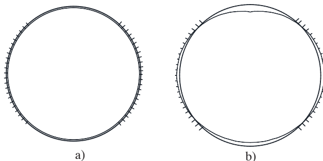
Fig. 14: Desplazamiento por compresi3n a) uniforme y b) no uniforme (ovalizaci3n).
