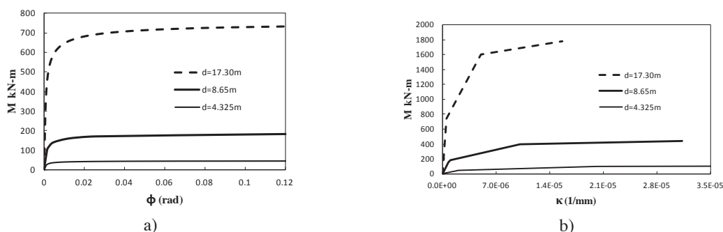
Fig. 12: Modelos constitutivos: a) M-φ en la junta longitudinal y b) M-κ en la junta continua.
