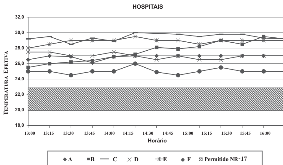
Figura 1 - Temperatura efetiva dos hospitais A, B, C, D, E e F obtida no primeiro dia de avaliação nos mesmos horários
