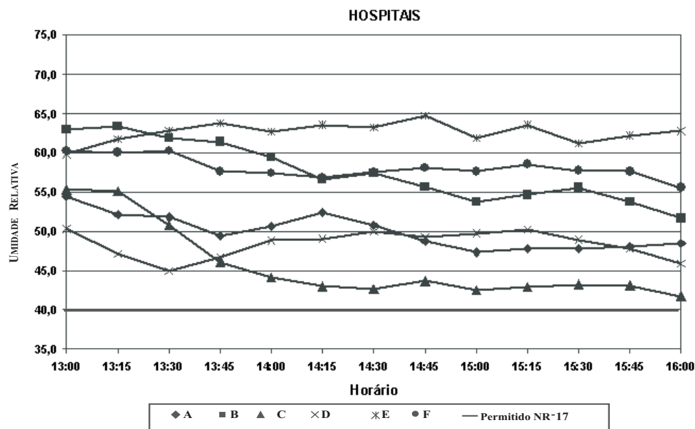
Figura 2 - Umidade relativa dos hospitais A, B, C, D, E e F obtida no primeiro dia de avaliação nos mesmos horários
