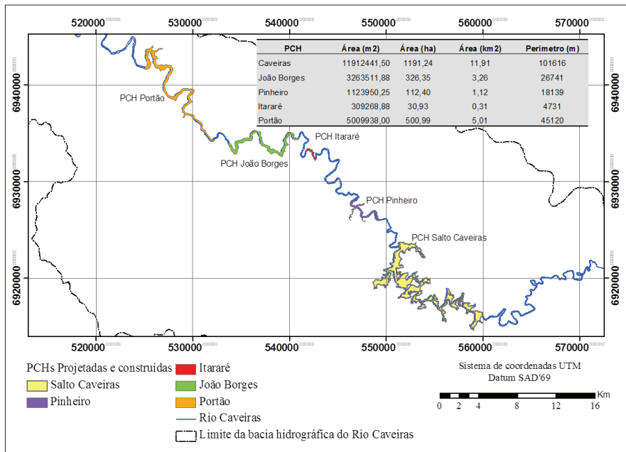
Figura 2 - Localização das PCHs Salto Caveiras (já construída), Pinheiro, Itararé, João Borges e Portão, ao longo do rio Caveiras.
