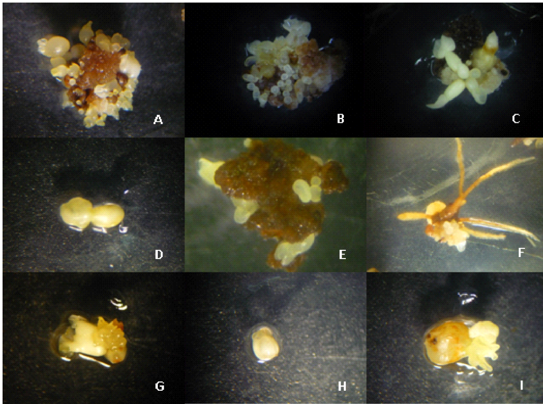
Figura 3. Embriogénesis somática en Theobroma cacao L. cv. 'SCA-6' A: Callo con estructuras embriogénicas de 'SCA-6' proveniente de un estaminodio subcultivado a 14 días. B: Callo con estructuras embriogénicas de 'SCA-6' proveniente de un pétalo subcultivado a 14 días. C y D: Detalle de embriones somáticos en etapa de torpedos. E: Callo con estructuras embriogénicas de 'SCA-6' subcultivado cada 28 días. F: Callo con respuesta embriogénica y presencia de raíces. G: Embriogénesis secundaria. H e I: Embriones deformes.
