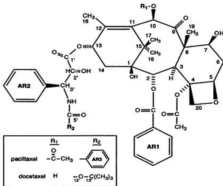
Figura 1. Estructura química del taxol. Modificado de: Nicolaou y Valiulin (2013).
