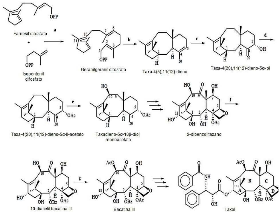
Figura 2. Esquema de la ruta de biosíntesis de taxol en Taxus spp. Las enzimas involucradas son geranylgeranil difosfato (a), taxadieno sintasa (b), citocromo P450 taxadieno 5 \alpha -hidroxilasa (c), taxa-4(20),11(12)-diene-5 \alpha -ol-O-acetiltransferasa (d), citocromo P450 taxano 10 \beta -hidroxilasa (e), taxano 2 \alpha -O-benzoiltransferasa (f), 10-diacetil baccatina III-10-O-acetiltransferasa (g) y pasos indefinidos múltiples (se indica en múltiples flechas). Modificado de: Walker y Croteau (2001).
