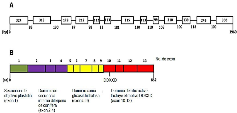
Figura 3. Estructura genómica y esquema de la estructura enzimática de taxadieno sintasa. A. Estructura genómica de taxadieno sintasa de Taxus baccata consistente de 13 exones (cajas) y 12 intrones (líneas); los números representan la longitud de los fragmentos en pares de bases (bp) B. Esquema de la estructura enzimática incluyendo la secuencia plastidial y las características principales de los motivos de terpeno sintasa, exones numerados (cajas) e intrones (líneas verticales) Tomado de: Trapp y Croteau (2001).
