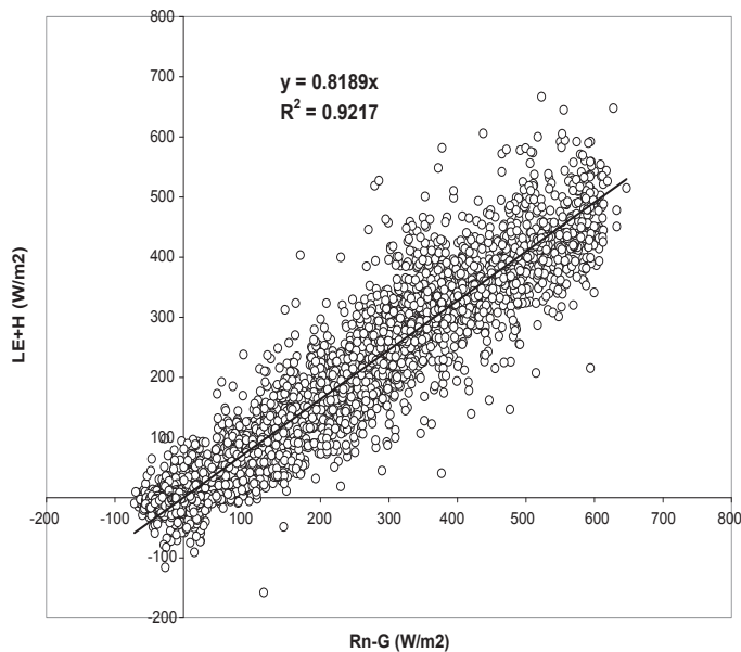
Figura 3. Energía disponible y flujos turbulentos a frecuencia de 30 min. en chile banana en el Valle del Yaqui, México. 2008.
