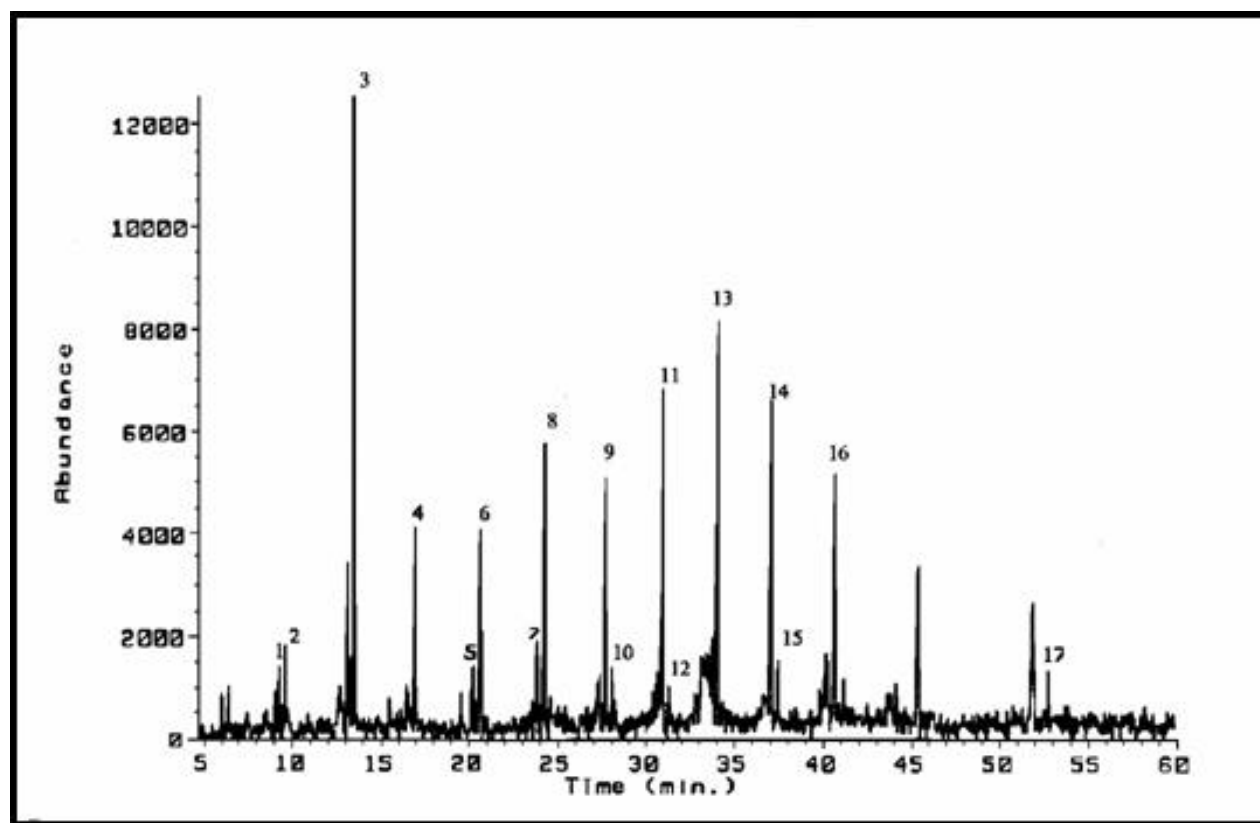
Fig. 7 Reaction Products Chromatogram (Ru/SiO 2 , 6% catalyst). 1) 1-pentadecanol, 2) Decycloxiolanol, 3) Octane, 4) Eicosane, 5) Pentadecanol (isomer), 6) Tetradecane, 7) 1-Heptadecanol, 8) Tetradecane (isomer), 9) Octane 2,4,6 – Trimetil, 10) Pentadecanol (isomer), 11) Hexadecane, 12) Heptadecanol (isomer), 13) Heptadecane, 14) Tetradecane (isomer), 15) Heptadecanol (isomer), 16) Octadecane, 17) Pentadecanol (isomer).
