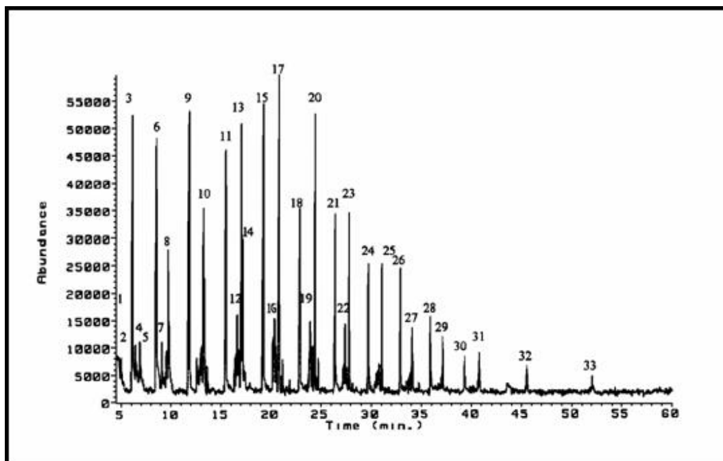
Fig. 8 Reaction Products Chromatogram (Fe/SiO 2 , 4% catalyst). 1) Hexanal, 2) Heptane, 3) 1-Pentanol, 4) Decanal, 5) Heptane (isomer), 6) 1-Pentene-2-Metil, 7) Nonane, 8) 1-Heptanol, 9) Dodecane, 10) 1-Octanol, 11) 5-Undecene, 12) Decane 2,3,5-Trimetil, 13) 1-Heptadecanol, 14) 1-Nonanol, 15) 5-Dodecene, 16) Heptadecane, 17) 1-Decanol, 18) 4-Nonene, 19) Tridecane, 20) Ciclohexane 1,2,3 -Trimetil, 21) 1-Octadecanol, 22) Heptadecane (isomer), 23) 1-Dodecene, 24) Tetradecane, 25) 9-Octadecene, 26) Heptadecane(isomer), 27) 1-Heptadecanol, 28) Heptadecane (isomer), 29) 1-Octadecanol, 30) Pentadecane, 31) Dodecane 1,1 Oxybis, 32) Ciclopentane 1-etil.
