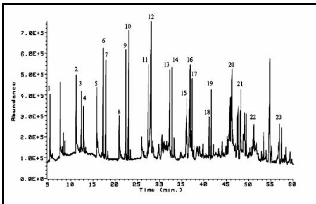
Fig. 9 Reaction Products Chromatogram (Fe/Ru/SiO 2 , 6,3%/ 5,5% catalyst). (*) 1) 1-Butanol, 2) 1-Butanol-3-metil, 3) Ciclopentane, 4) Nonane, 5) 1-Heptanol, 6) 1-Octanol, 7) Tetradecane, 8) 1-Octanol, 9) Ciclooctane, 10) Undecane, 11) Ciclobutane 1-butil 2-etil, 12) Dodecane, 13) 5-Tetradecene, 14) Heptadecane, 15) Bencen propanoic acid, 16) Propanedioic acid, 17) Heptadecane (isomer), 18) Tetradecane(isomer), 19) Hexadecane, 20) Heptacosane, 21) Pentadecane, 22) Decane 6-etil, 2-metil, 23) Tridecane.
